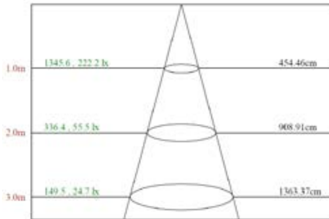
Max. Avr Beam angle of C150 plusse 152-49
